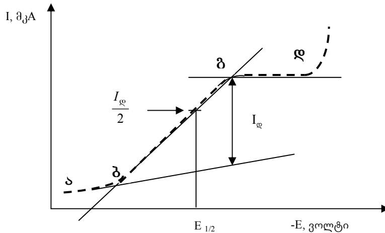
ნახ. 6.4.2. ტიპური პოლაროგრამა
