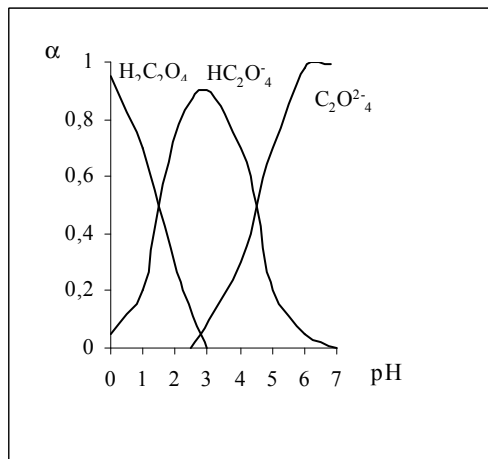
ნახ. 7.1.1. მჟაუნმჟავას წონასწორული ფორმების განაწილების დიაგრამა
