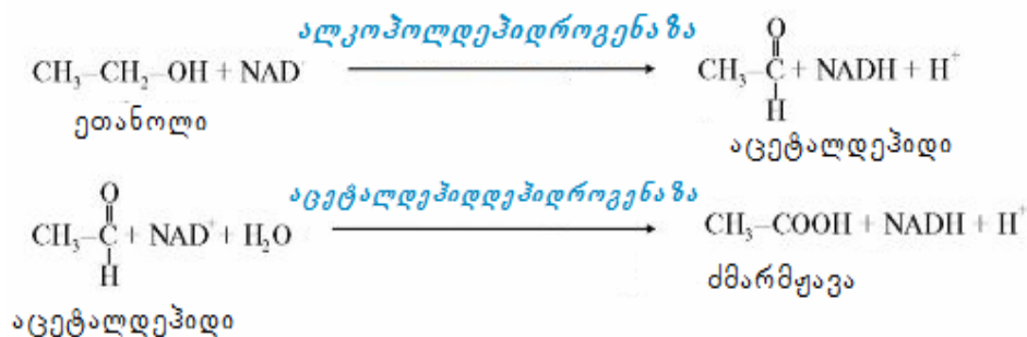
სურათი VIII.39. ეთანოლის დაქანგვა NAD-დამოკიდებული დეჰიდროგენაზებით
